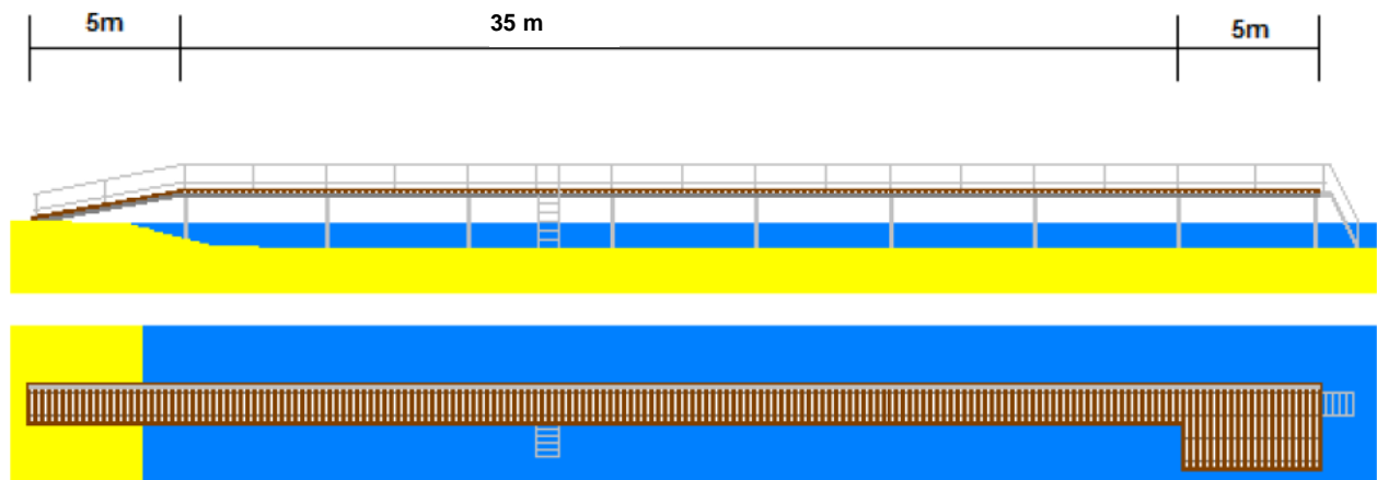
Skitse EB badebro, 45 m lang, 1,6 m bred, platform på de yderste 5 m er 3,5 m bred.
